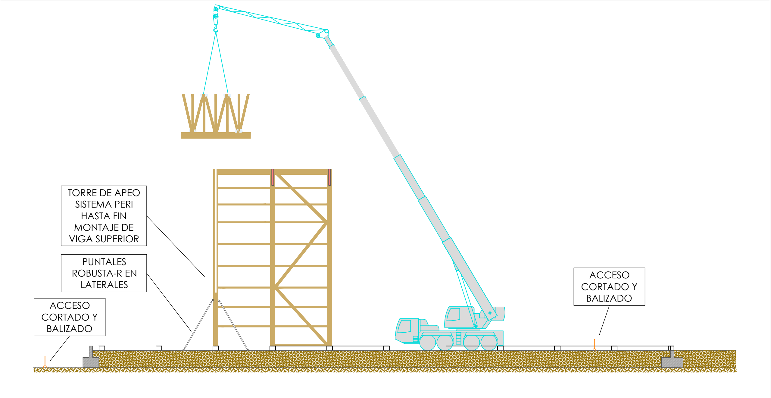
Montaje de pórticos de nave y celosías (fases 1.c a 1.h) - sección longitudinal
