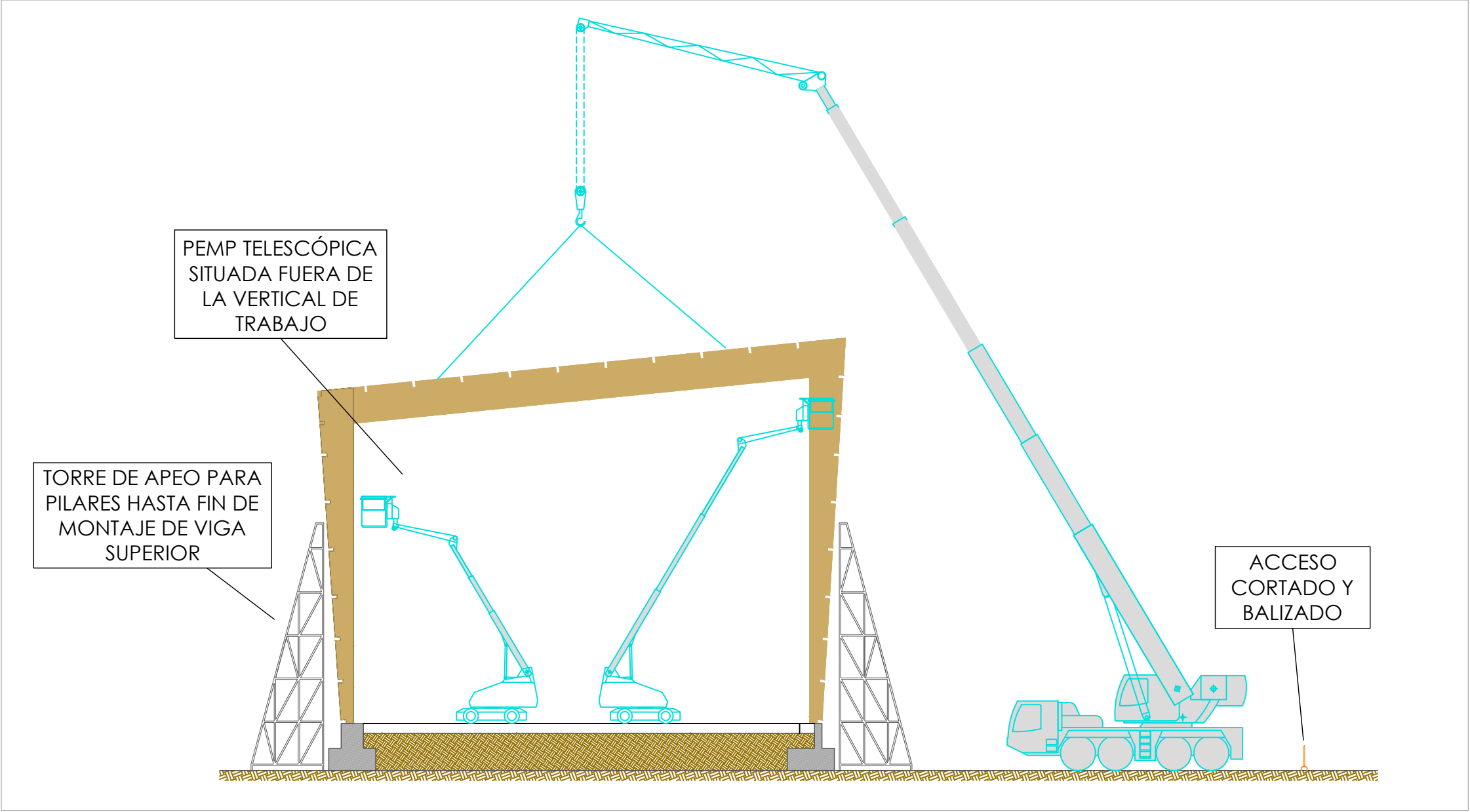
Montaje de pórticos de nave y celosías (fases 1.c a 1.h) - sección transversal
