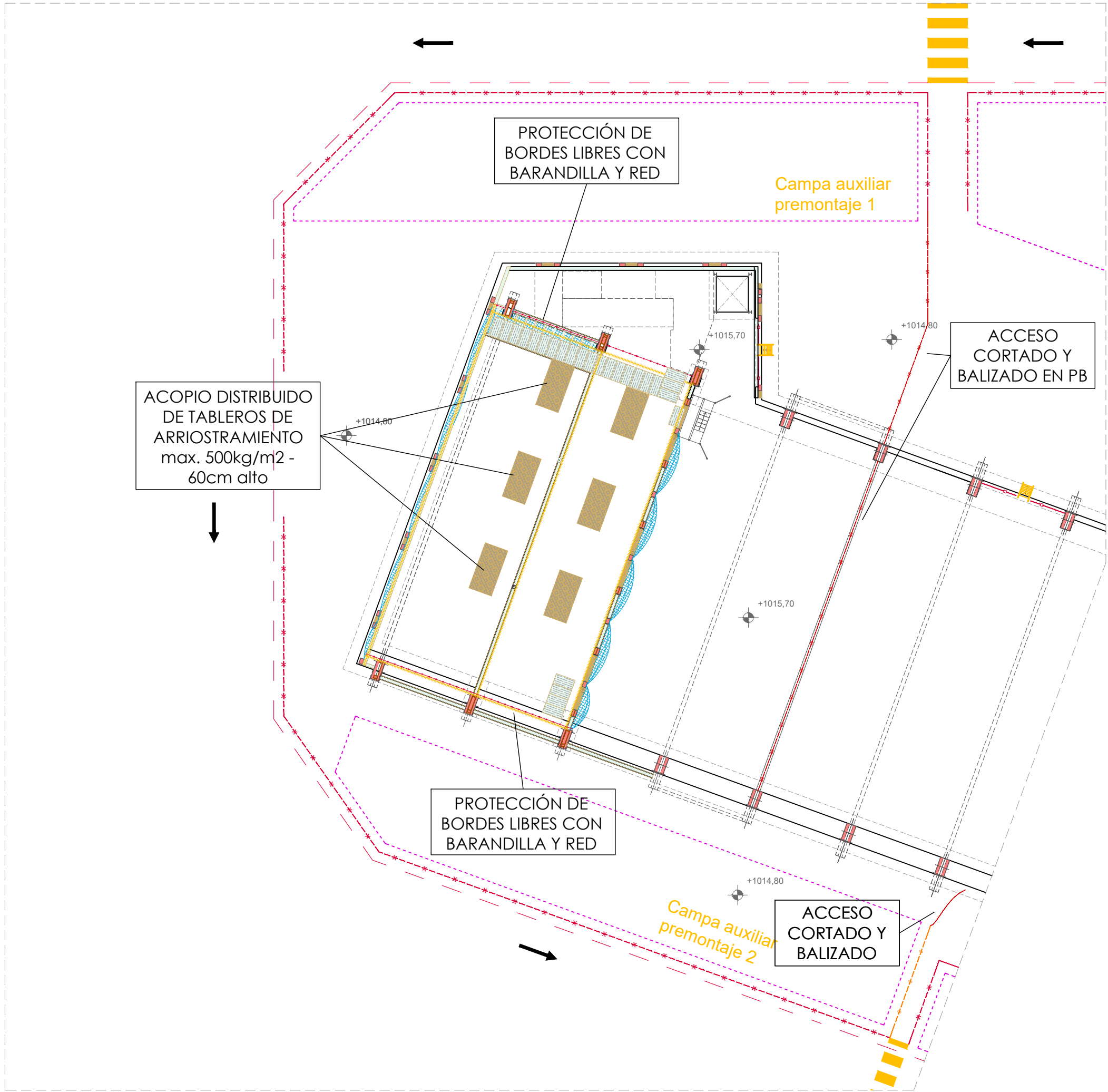
Montaje de módulos de forjado en planta tipo y acopio de paneles de arriostramiento (II)
