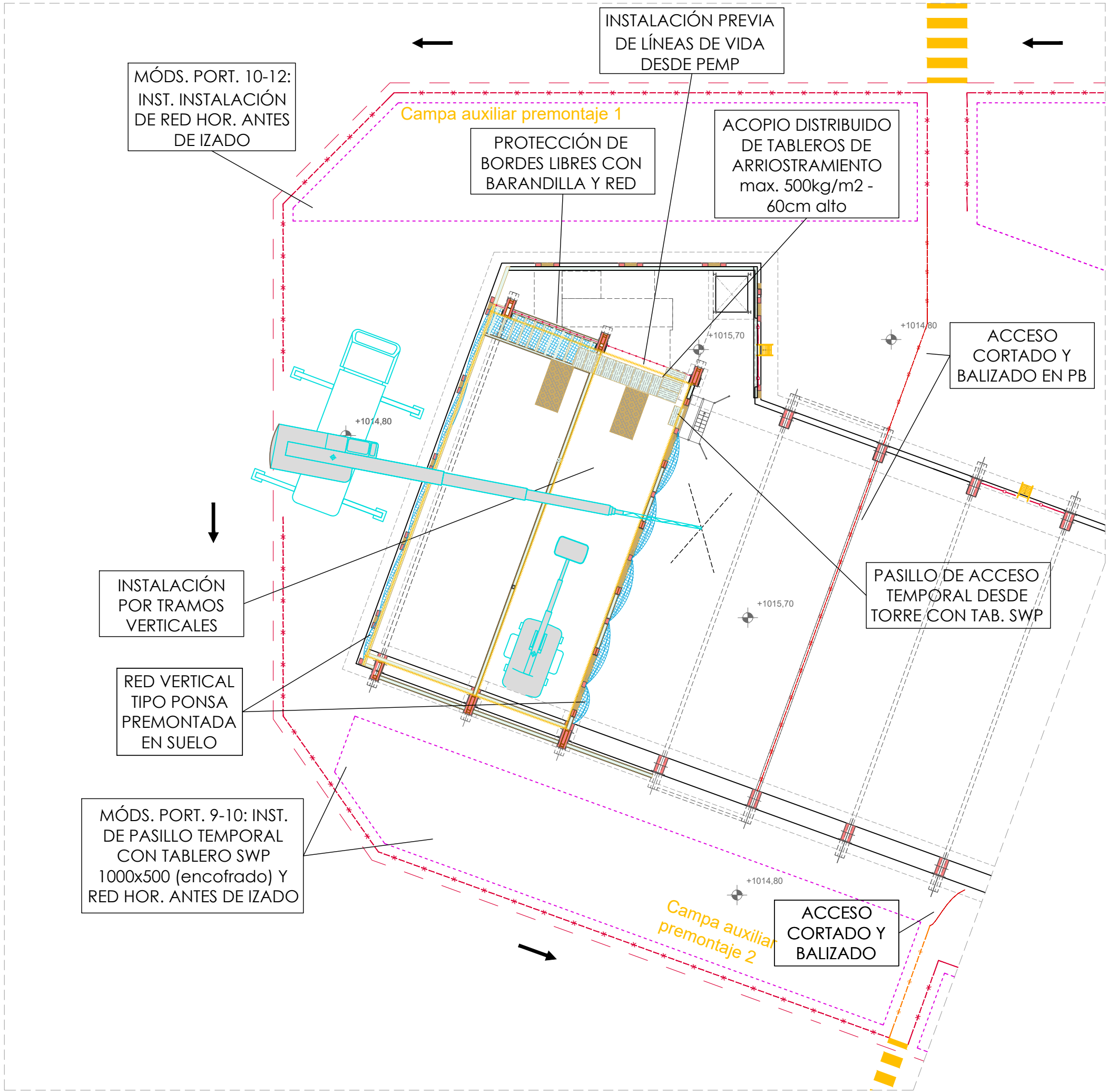
Montaje de módulos de forjado en planta tipo y acopio de paneles de arriostramiento (I)
